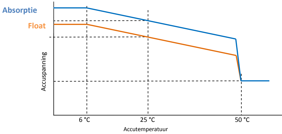
Afbeelding 1: temperatuurcompensatiecurve
