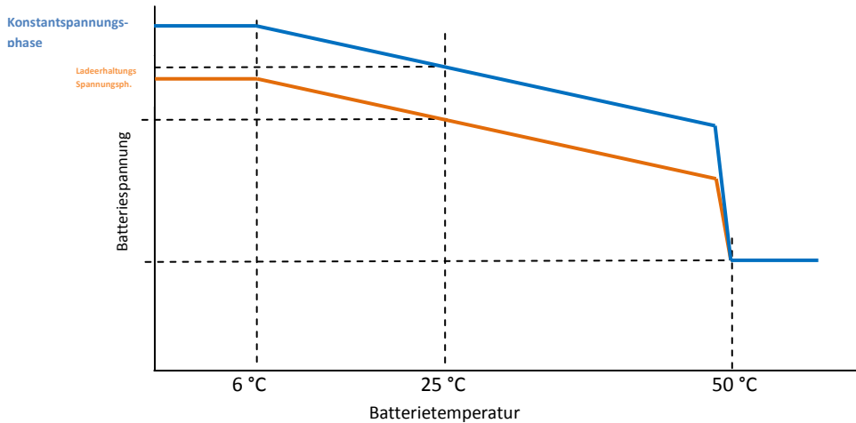
Abbildung 1: Temperaturkompensationskurve
